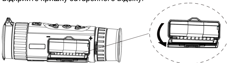
Рисунок 2-2 Відкриття кришки батарейного відсіку
