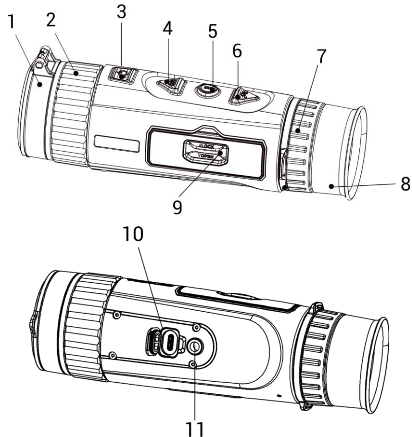
Рисунок 1-1 Зовнішній вигляд
