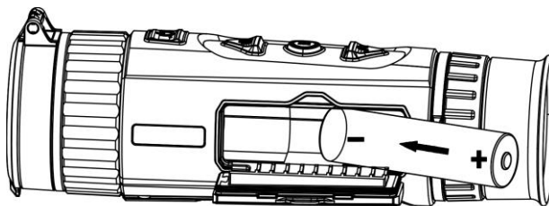
Рисунок 2-3 Установлення батареї
