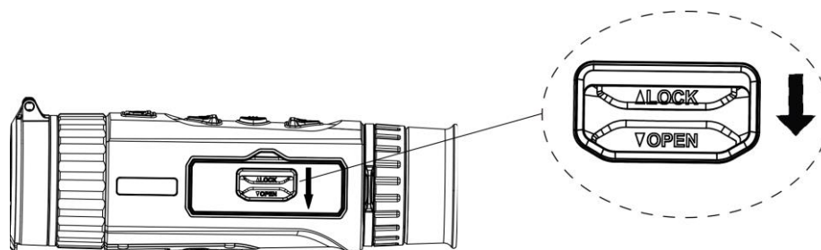
Рисунок 2-1 Розблокування кришки батарейного відсіку
