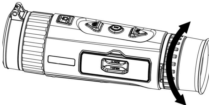
Рисунок 3-1 Регулювання діоптрій
